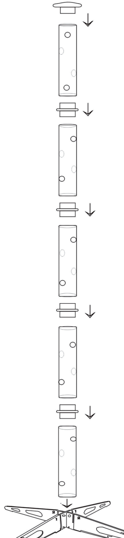
Plaats de tubes met tussenringen op de bodemstandaard
