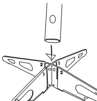
Plaats de tubes met tussenringen op de bodemstandaard
